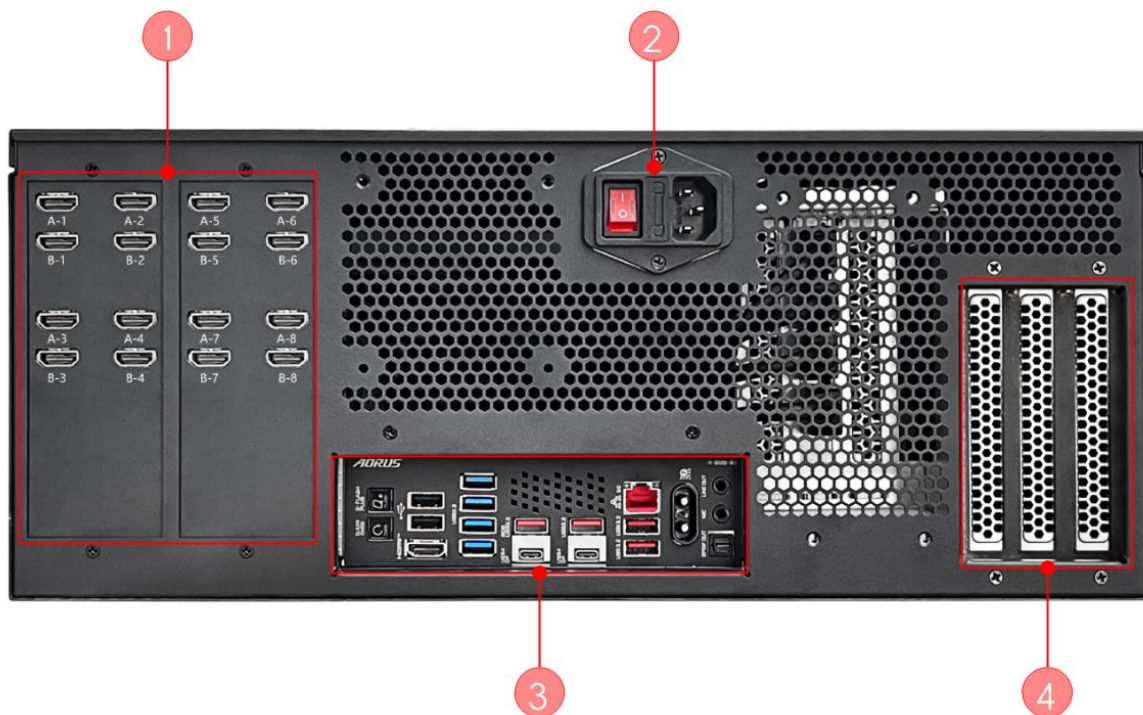
后面板
